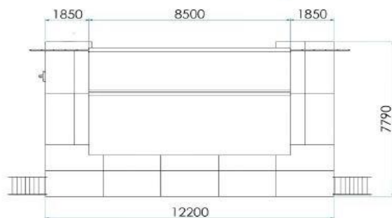
Escenario Móvil desplegado Vista Planta
