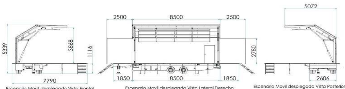
Escenario Móvil desplegado Vista Frontal
