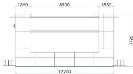
Escenario Móvil desplegado Vista Planta
